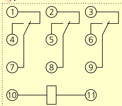
Реле РП53 с 3-мя переключающими контактами
