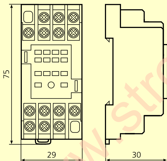
Розетка PYF14A для реле РП54 с 4-мя переключающими контактами
