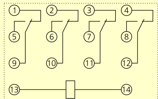
Реле РП54 с 4-мя переключающими контактами
