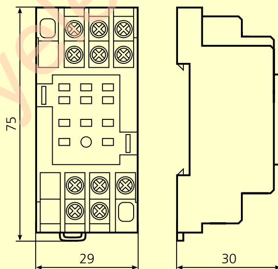
Розетка PYF11A для реле РП53 с 3-мя переключающими контактами
